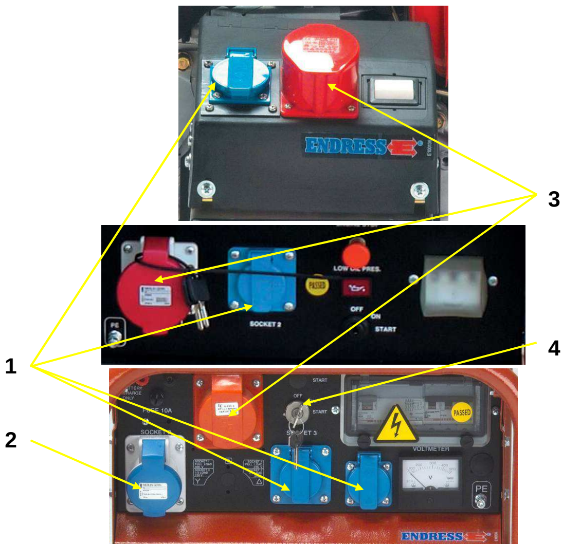
Рис. 4.4: Подключение потребителей
