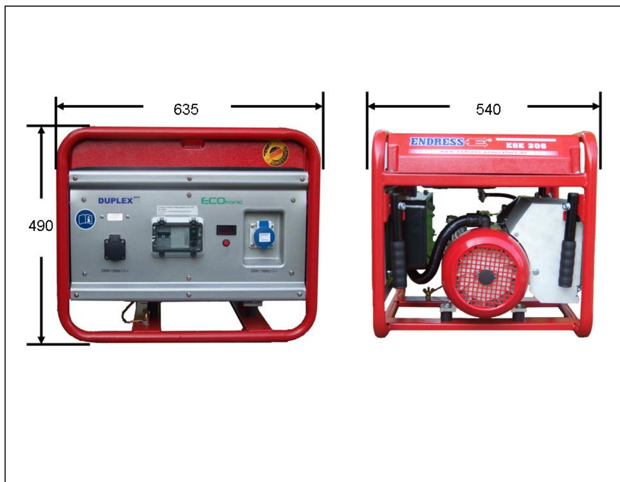
Рис. 7-1: Габариты электростанции (306 SG-GT Duplex)
